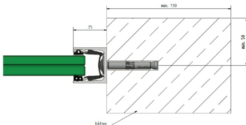
Représentation d'un exemple de fixation du profil au gros-œuvre
