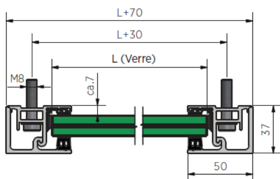
Représentation d'un exemple de fixation du profil à un cadre en aluminium
