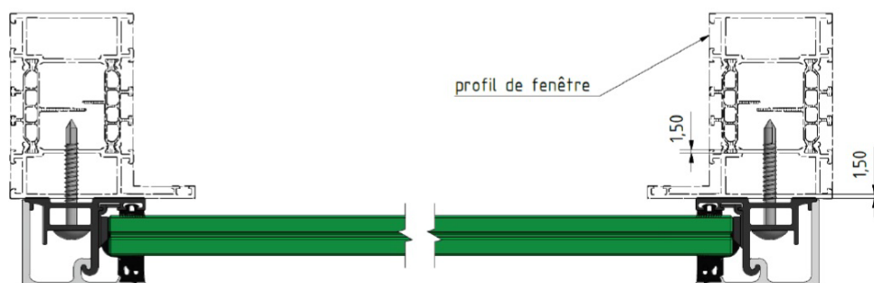
Représentation d'un exemple de fixation du profil à un cadre en aluminium
