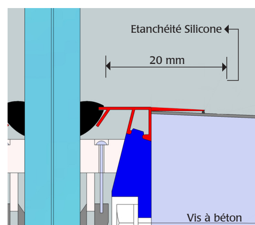
■ Couvertine GARDA 1 AY
