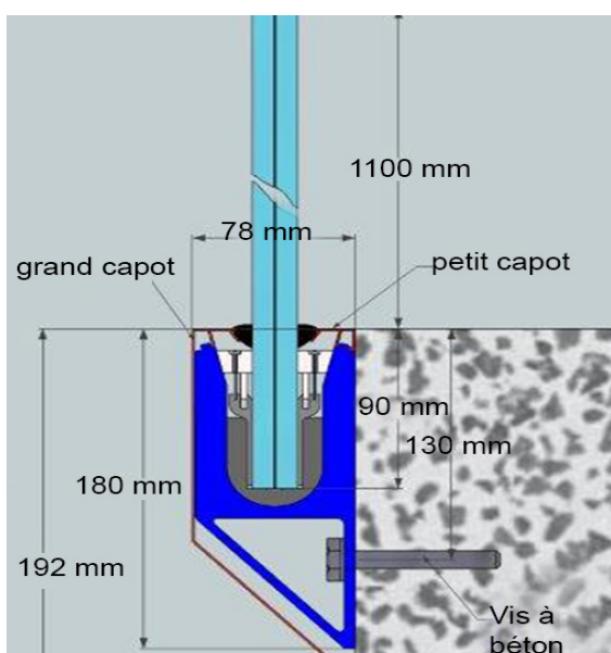
■ Garde-corps sur profil GARDA 1 AY
