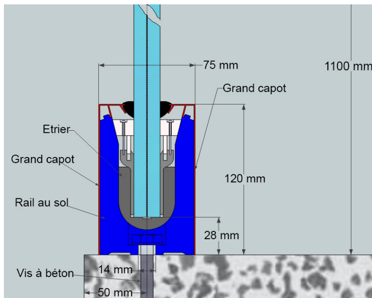
Garde-corps sur profil GARDA 1 F
