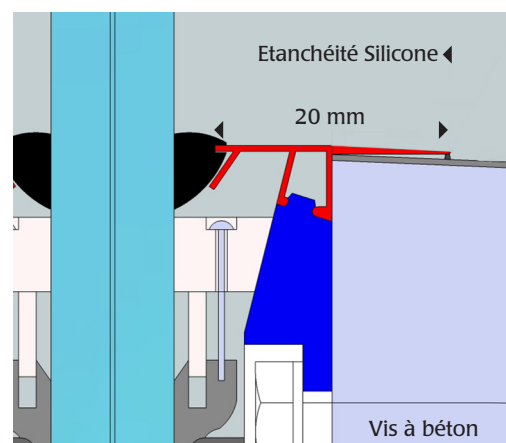
Couvertine GARDA 1 A
