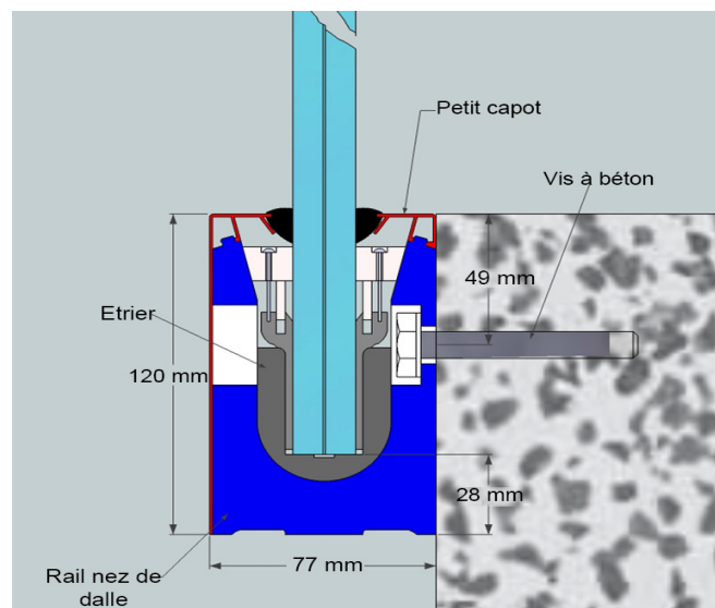
Garde-corps sur profil GARDA 1 A
