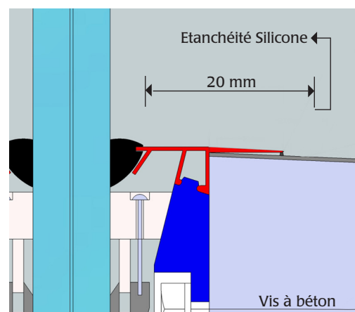
Couvertine GARDA 1 FE
