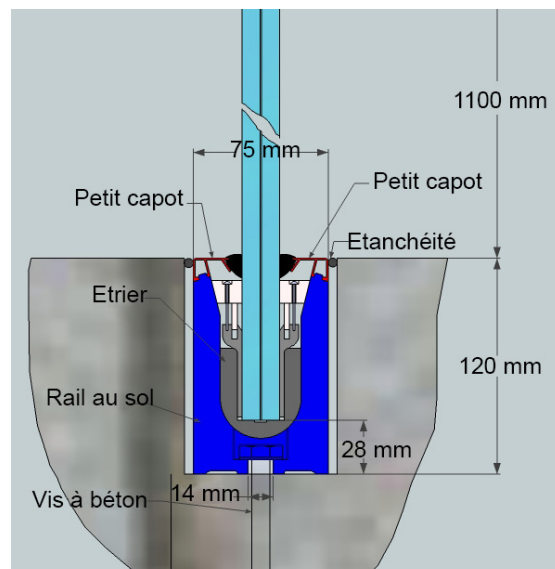
Garde-corps sur profil GARDA 1 FE
