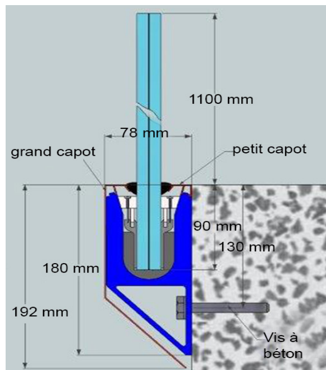
Garde-corps sur profil GARDA 1 AY
